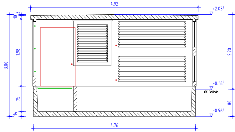
Schnitt A-A
