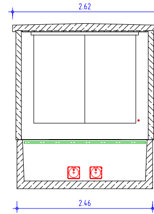
Schnitt B-B
